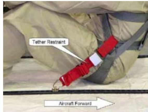
Figura 7. Fijación de sujeción de la correa al piso para asientos de piso orientados hacia atrás
